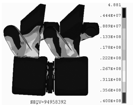
Рисунок 10 – Напряженное состояние модели с протезом, контактная задача
