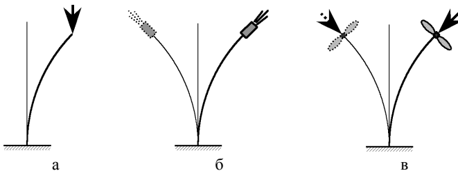
Рисунок 1 – Схема нагружения трубы продольными силами
