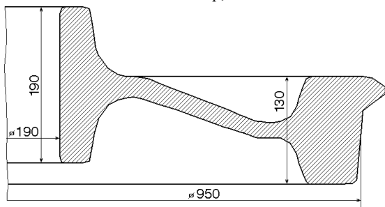
Рис. 2. Стандартное цельнокатаное вагонное колесо
