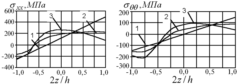
Эпюры напряжений в сечении цилиндра
