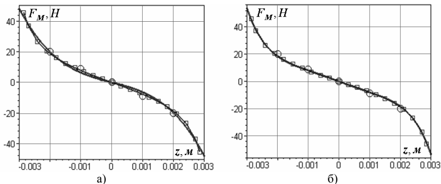
Рисунок 4 – Зависимость магнитной силы от аксиального смещения ротора (○ – экспериментальные и □ – расчетные данные): а) аппроксимация кубическим полиномом, б) аппроксимация полиномом пятой степени
