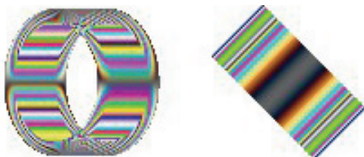
Рисунок 1 – Вид плосконапряженного цилиндрического тела в скрещенных поляриодах, повернутое вокруг оси Y, на угол 45^\circ , и вид с торца
