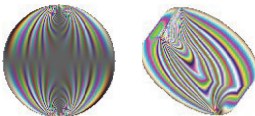
Рисунок 2 – Вид плосконапряженного диска в скрещенных поляриодах, перпендикулярно поверхности и под углом
