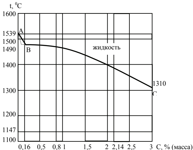
Рисунок 1 – Диаграмма железо-углерод: АВ – (линия ликвидус) показывает температуру начала кристаллизации \delta -феррита из жидкого сплава; ВС – (линия ликвидус) соответствует температуре начала кристаллизации аустенита.
