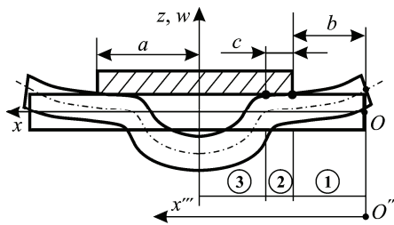
Рисунок 2 – Характерная картина распределения прогибов оболочки и контактных зон на фиксированной конфигурации контакта с одной зоной отрыва: 1 – свободный участок оболочки; 2 – зона термоупругого контакта цилиндрической оболочки с бандажом; 3 – зона отрыва
