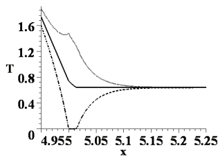
Рисунок 5 – Распределение температуры (°С) в оболочке в области контакта вдоль оси x (м): серая линия (верхняя) – внутренняя поверхность, черная линия (средняя) – средняя поверхность, пунктирная линия (нижняя) – внешняя поверхность
