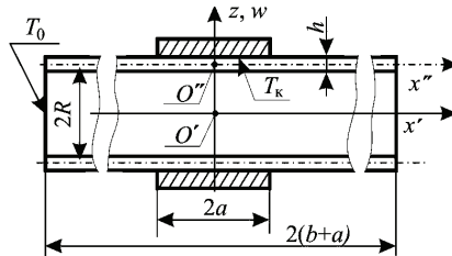
Рисунок 1 – Расчетная схема задачи о термоупругом контакте цилиндрической оболочки с бандажом
