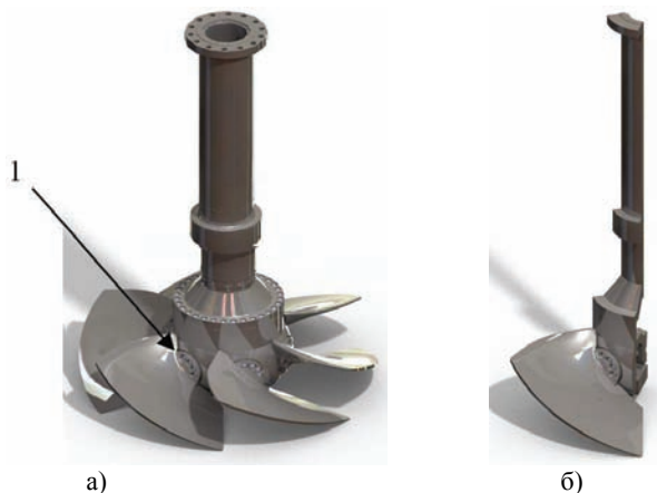
Рисунок 1 — Конструкция колеса гидротурбины с ротором: а) целая часть, б) циклически симметричная часть
