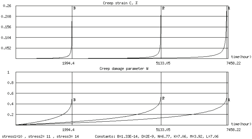
Криві повзучості та пошкоджуваності
