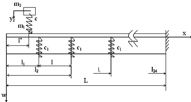
Рисунок 2 – Система «вагон – рейка на проміжних пружних опорах»
