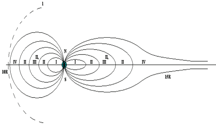
Рисунок 1 – Радіаційний пояс Землі: 1 – границя магнітосфери; I – внутрішній (протонний) пояс; II – пояс протонів малих енергій; III – зовнішній (електронний) пояс; IV – зона квазі-захвату часток сонячного вітру. Переріз відповідає полуденному меридіану
