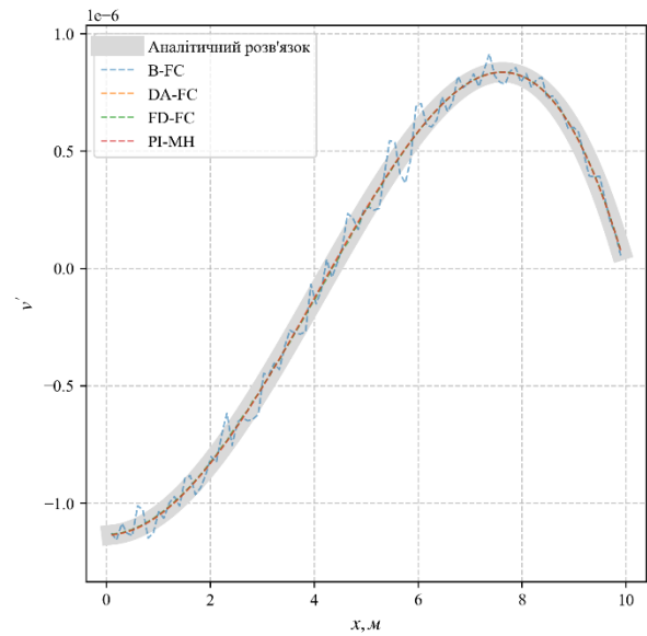
Рис. 10 – Перша похідна 3:1 (0.5)
