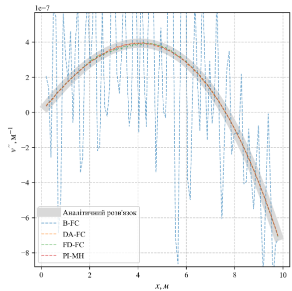
Рис. 12 – Друга похідна 3:1 (0.5)
