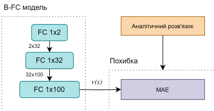
Рис. 1 – Архітектура базової повнозв’язної моделі B-FC.
