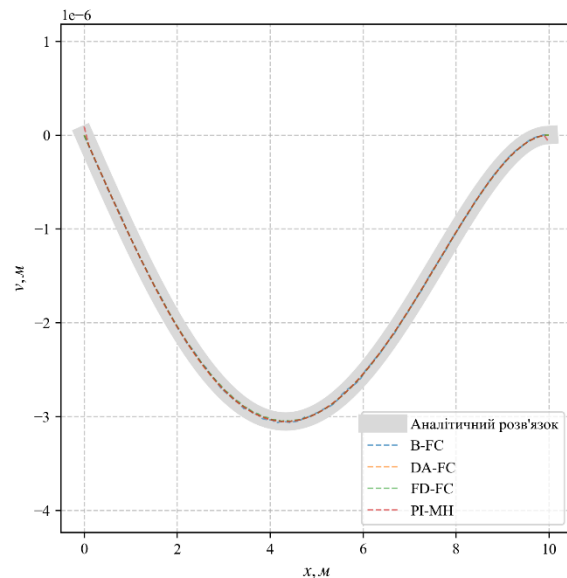
Рис. 8 – Прогин 3:1 (0.5)
