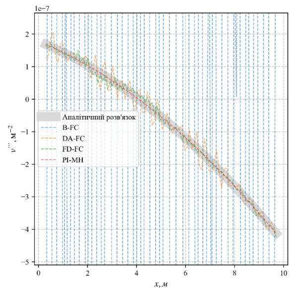
Рис. 14 – Третя похідна 3:1 (0.5)
