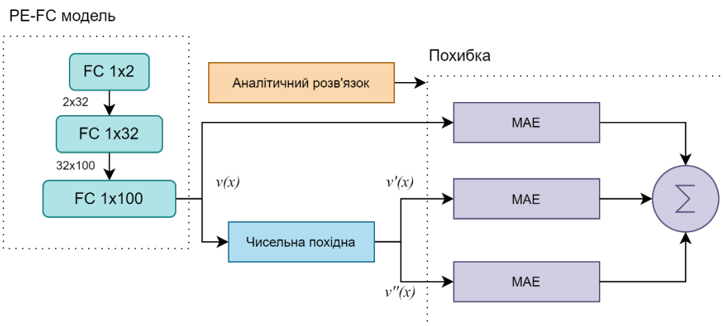
Рис. 2 – Архітектура повнозв’язної моделі з фізичною функцією втрат PE-FC.
