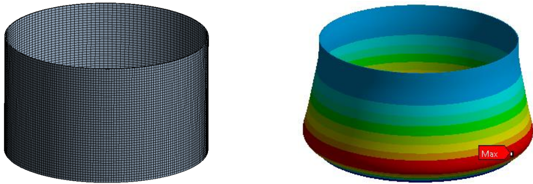
Рис. 2 – Скінченно-елементна модель бака
