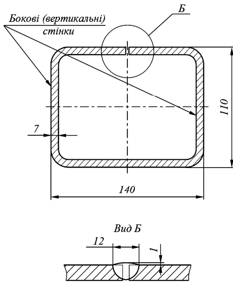
Рисунок 3 – Поперечний переріз верхнього обв'язування
