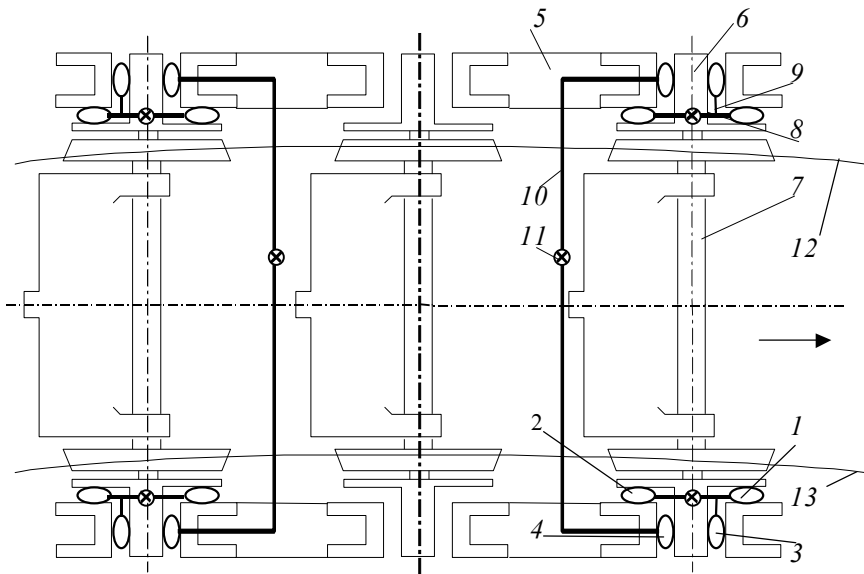
Схема устройства для РУКП на базе гидравлических цилиндров: 1, 2 – поперечные гидравлические цилиндры; 3, 4 – продольные гидравлические цилиндры; 5 – рама тележки; 6 – буksа; 7 – колесно-моторный блок; 8, 9, 10 – трубопроводы; 11 – дроссель; 12, 13 – наружный и внутренний рельсы кривой.
