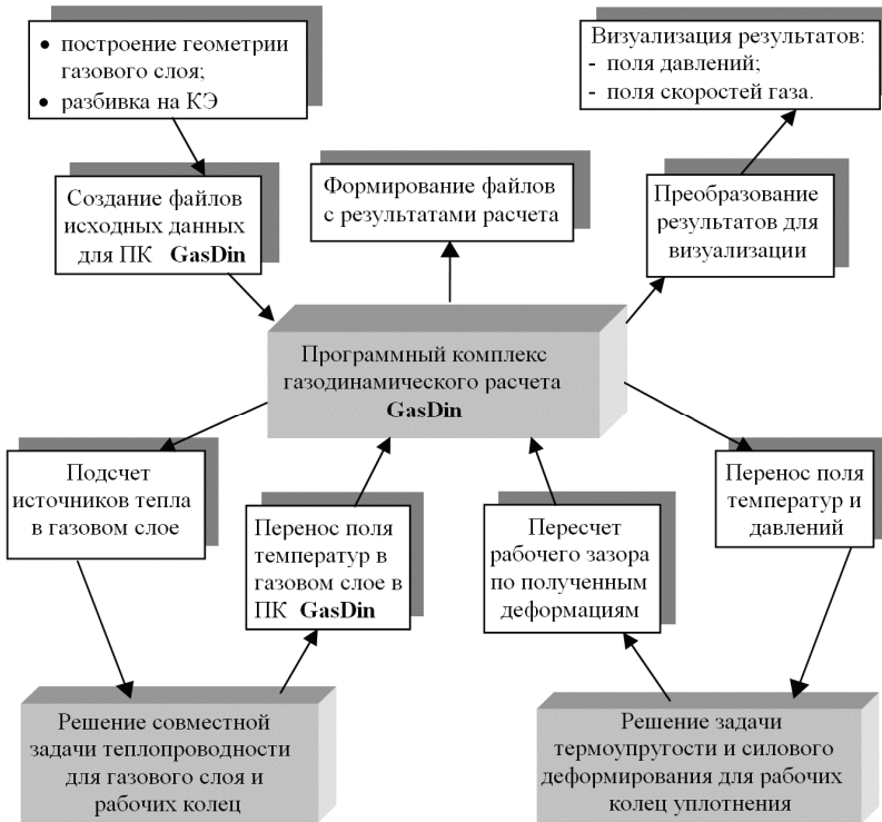
Рисунок 2 – Блок-схема программной реализации алгоритма решения
